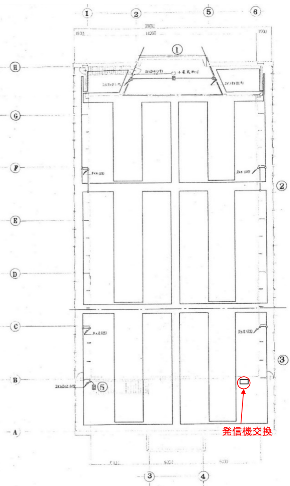
体育館 2階平面図
