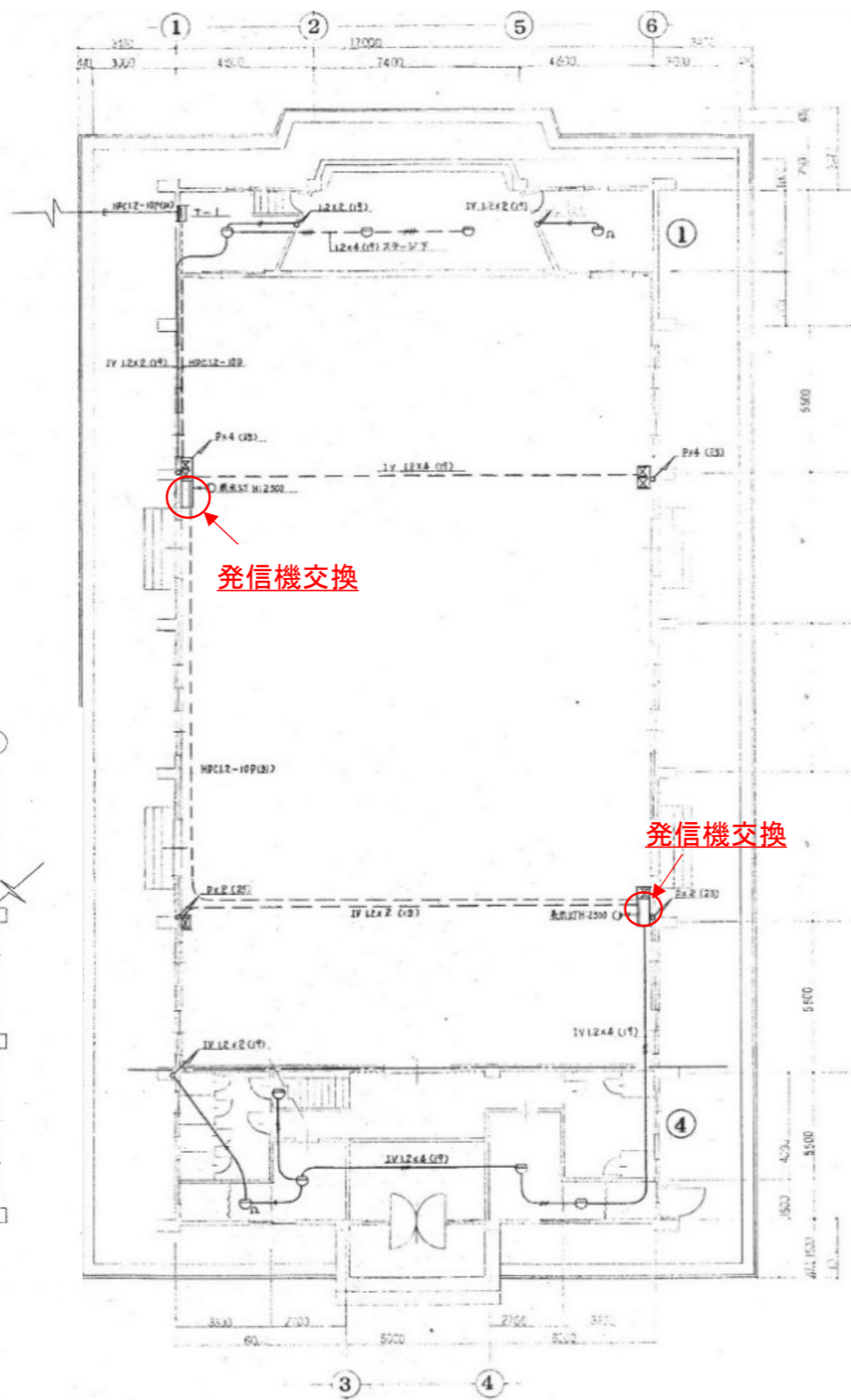
体育館 1階平面図
